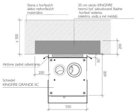
Schéma zabudovania pred stenou hr. max. 500 mm
