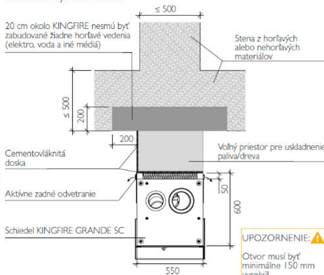
Schéma zabudovania ako deliaci prvok priestoru so skladovacím priestorom na drevo pred stenou s hrúbkou viac ako 50 cm a s nadväzujúcou stenou
