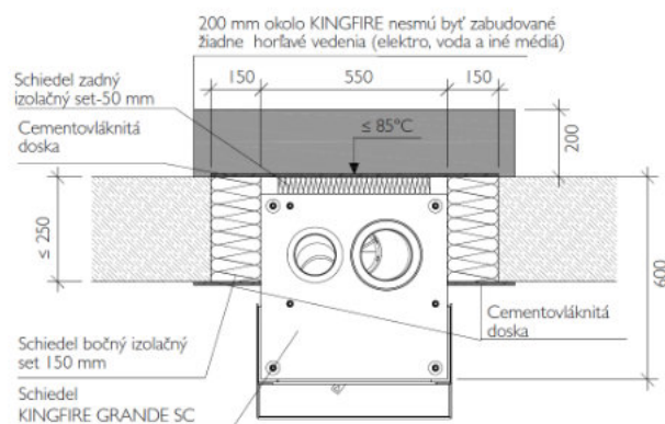
Schéma zabudovania v stene hrúbky max. 25 cm
