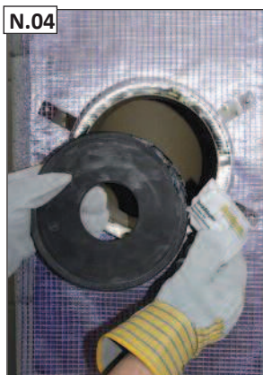
Palei visą kišamojo adapterio kontūrą užtepkite lubrikanto.
