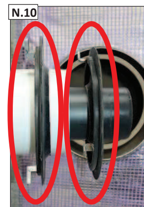
Sumontuotas jungiamasis vamzdis turi būti prakištas kiaurai pro kišamąjį adapterį.
