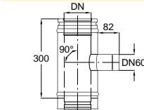
T-idom 90 fokos 60 mm-es csatlakozással
