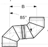
Könyök 85° ábra
