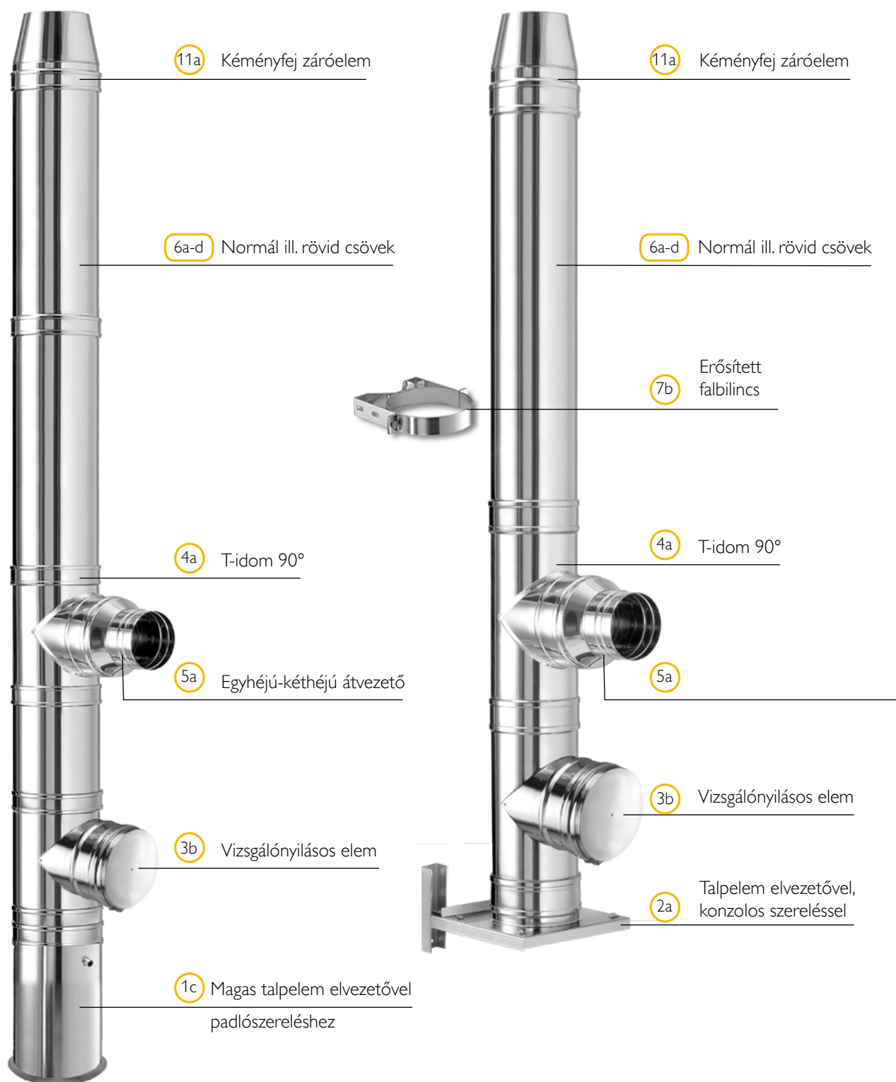
Padlószerelés
