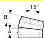
Könyök 15 fokos
