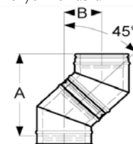
Könyök 45° ábra
