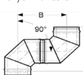
Könyök 90° ábra
