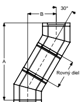
Könyök 30° csőelemmel
