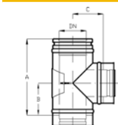
T-idom 90 fokos vizsgáló nyílással (kör alakú)
