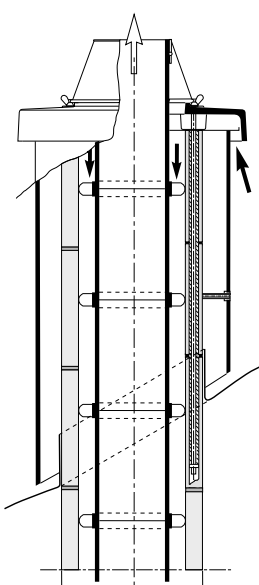
Hőszigetelt, vakolt fejkialakítás
