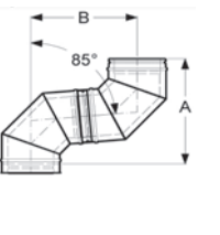
Könyök 90° ábra
