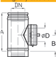
Vizsgálónyílásos elem N1 (rövid)
