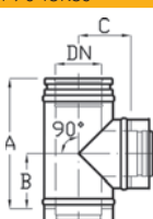
T-idom 90 fokos
