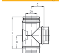
T-idom 90 fokos vizsgáló nyílással (köralakú)
