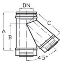
T-idom 45 fokos
