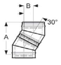
Könyök 45° ábra
