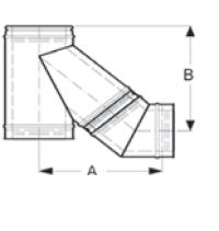
T-idom 45°és könyök 45° ábra
