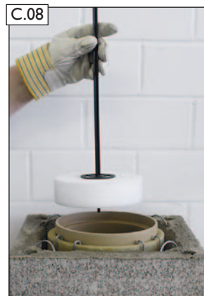
RAPID-Fugendichtreste mit Fugenglätter abstreifen.
