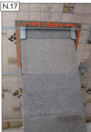
N.17 Fertigansicht mit ausge-dämmtem Dachdurchgang gem. FeuVo der Länder.
