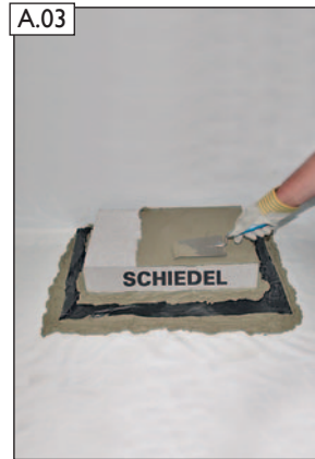
A.03 Mörtelbettauflage bei ergänzender Verwendung der Thermofußplatte (nicht im Lieferumfang enthalten).
