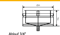
HDW WT – Kondensatschale
