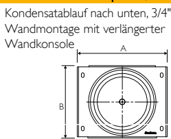
HDW WT – Stützplatte
