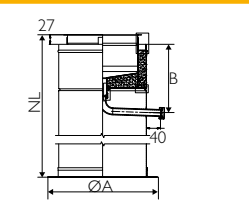
HDW WT Grundplatte, Ablauf unten
