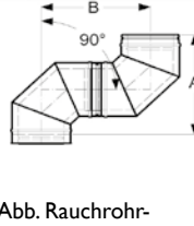
Abb. Bogen 90°
