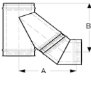
Abb. Rauchrohr- anschluss 45° mit Bogen 45°
