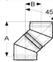
Abb. Bogen 85°
