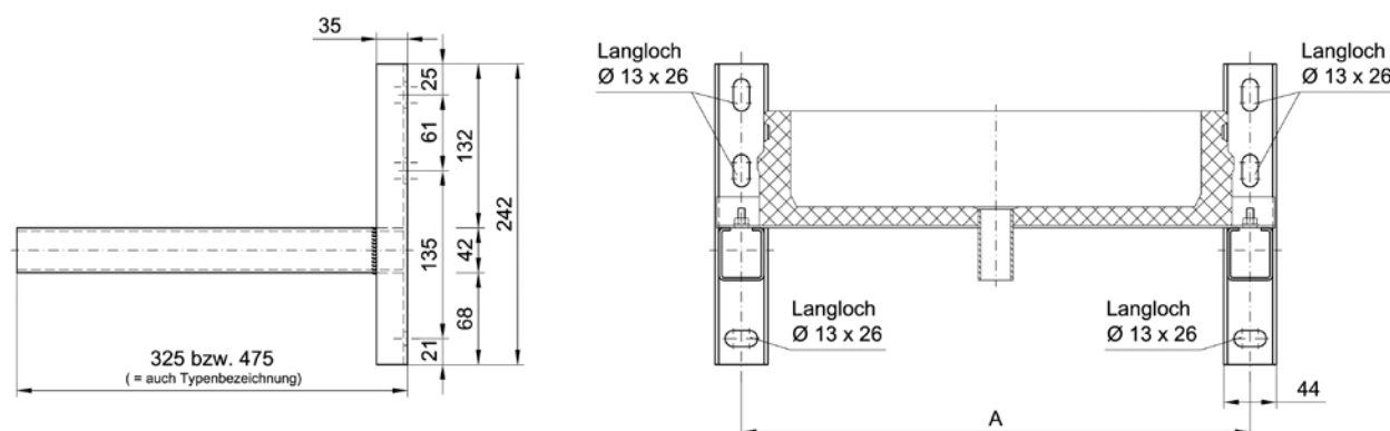
Montagemaße Wandmontage bei Typ 570 bis Typ 1304
