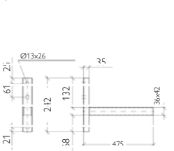
Verlängerte Wandkonsole (Paar)*
