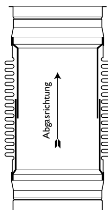
Senkrechter Einbau
