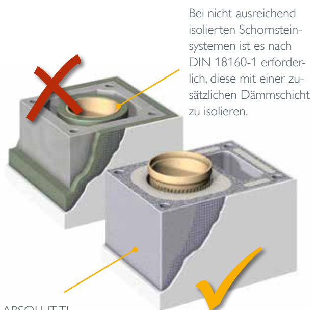
ABSOLUT TL mit werkseitig gedämmtem Compound-Mantelstein mit Thermo-Luftzug.
