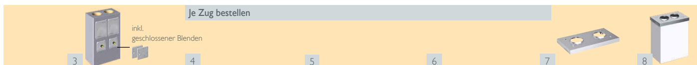
3 Fertigfuß 4) Höhe 107 cm 4 Fertigfußpaket 5 Anschlusspaket RA 90° 6 Anschlusspaket PA oberer Putztüranschluss 7 Edelstahl-Zuluftkopfplatte 8,5 cm Überstand 8 Kaminkopf Höhe 150 cm
