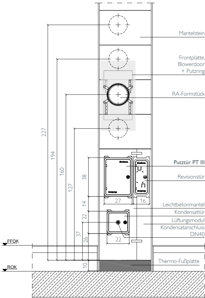
Standard Fertigfuß Anschluss Höhen
