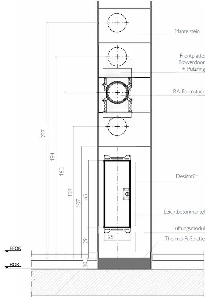
Fertigfuß mit Designtür Anschluss Höhen
