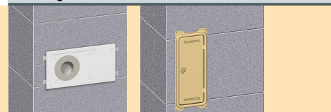
LAS Zuluft-Adapter 7) für Thermo-Luftzug, Anschluss Längsseite
