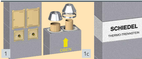
PARAT-Set 2) für Fußteil und Mündung
