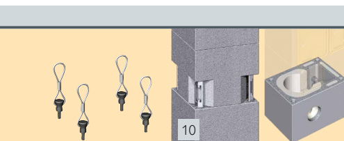
10 Versetzschaufen 9) Set: 4 Stück, SRd 12
