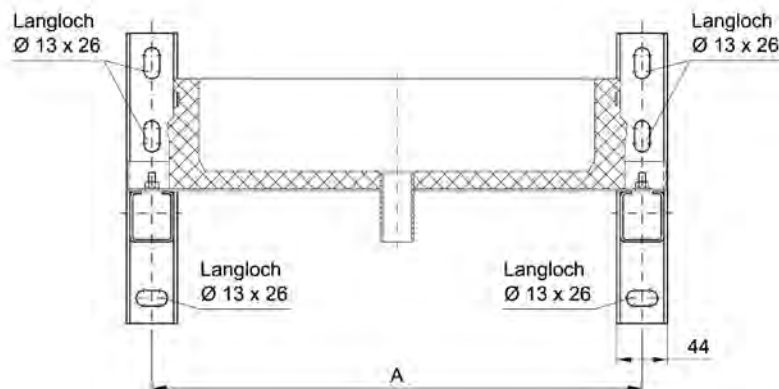
Montagemaße Wandmontage bei "Montageschiene" Typ 325 und Typ 475
