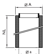
Schachtelement 1000 Frontplatte abnehmbar
