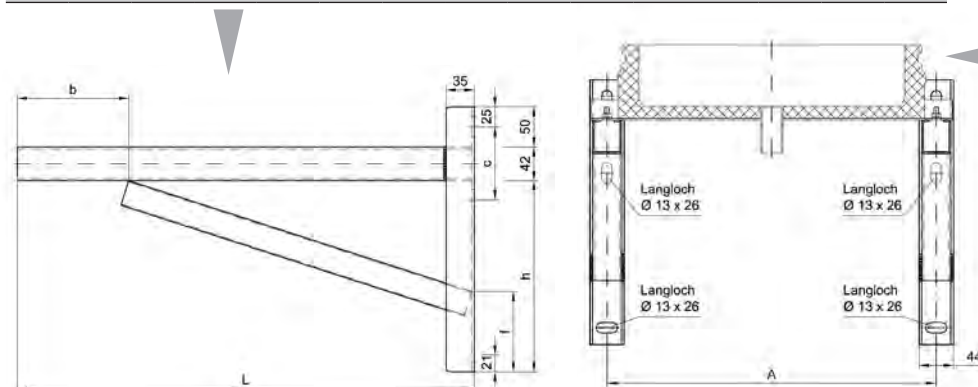
Montagemaße Wandmontage bei "Montageschiene" Typ 570 bis Typ 1504
