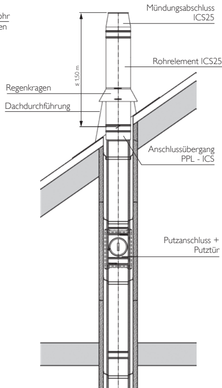
Systemdarstellung PRIMA PLUS
