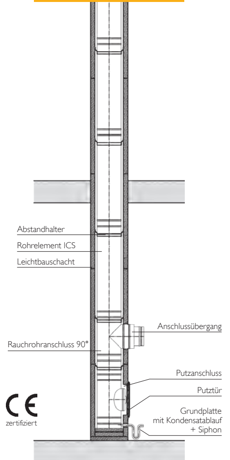
Systemdarstellung ICS
