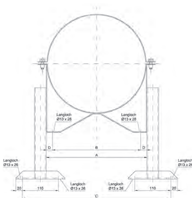
Montagemaße bei Wandhalter inkl. Verlängerungen L1 - L4; L7, L8
