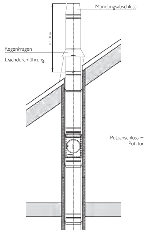
Systemdarstellung ICS
