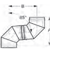
Abb. Bogen 85°
