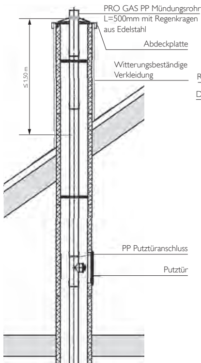
Systemdarstellung PRO GAS PP
