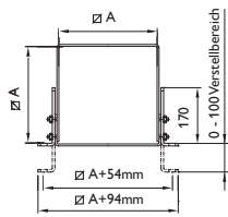
Sparrenhalter (Einzelteile, Aluwinkel lose gepackt)
