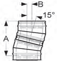
Abb. Bogen 30°
