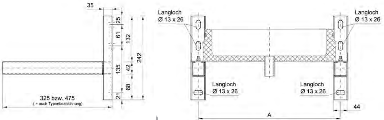
Montagemaße Wandmontage bei "Montageschiene" Typ 475
