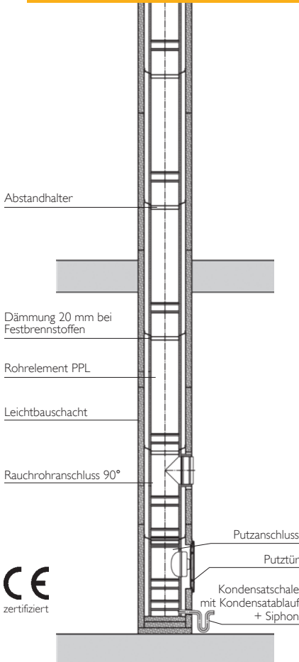
Systemdarstellung PRIMA PLUS
