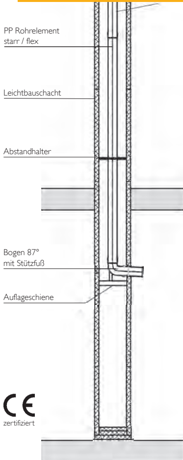
Systemdarstellung PRO GAS PP
