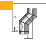
Úhyb 45° (s použitím kolena s kontrolním otvorem)
