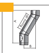
Úhyb 30° s rovnými díly a s použitím kolena s kontrolním otvorem
