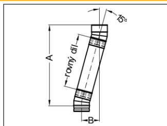
Délka úhybu (B) při použití kolen 15° a rovných dílů
