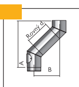
Úhyb 45° s rovnými díly a s použitím kolena s kontrolním otvorem
