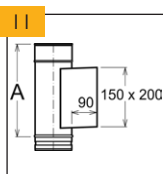
Dviřkový díl s vnitřními dviřky 150 x 200 (Dviřkový_díl)
