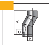
Úhyb 30° (s použitím kolena s kontrolním otvorem)
