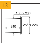
Dviřka s prodloužením (Dviřka_140x200_s_pr)
