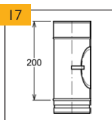
Díl s KO pro podtlak (Díl_s_KO_zápl.)
